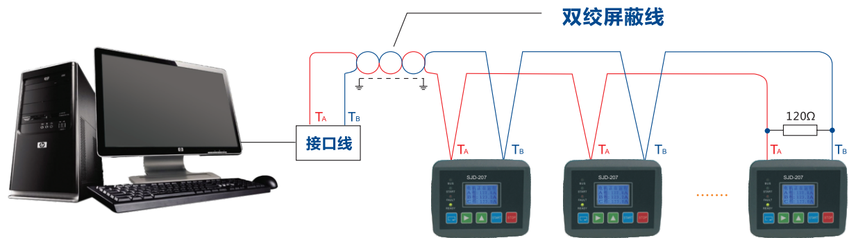
图14 计算机通讯连接
