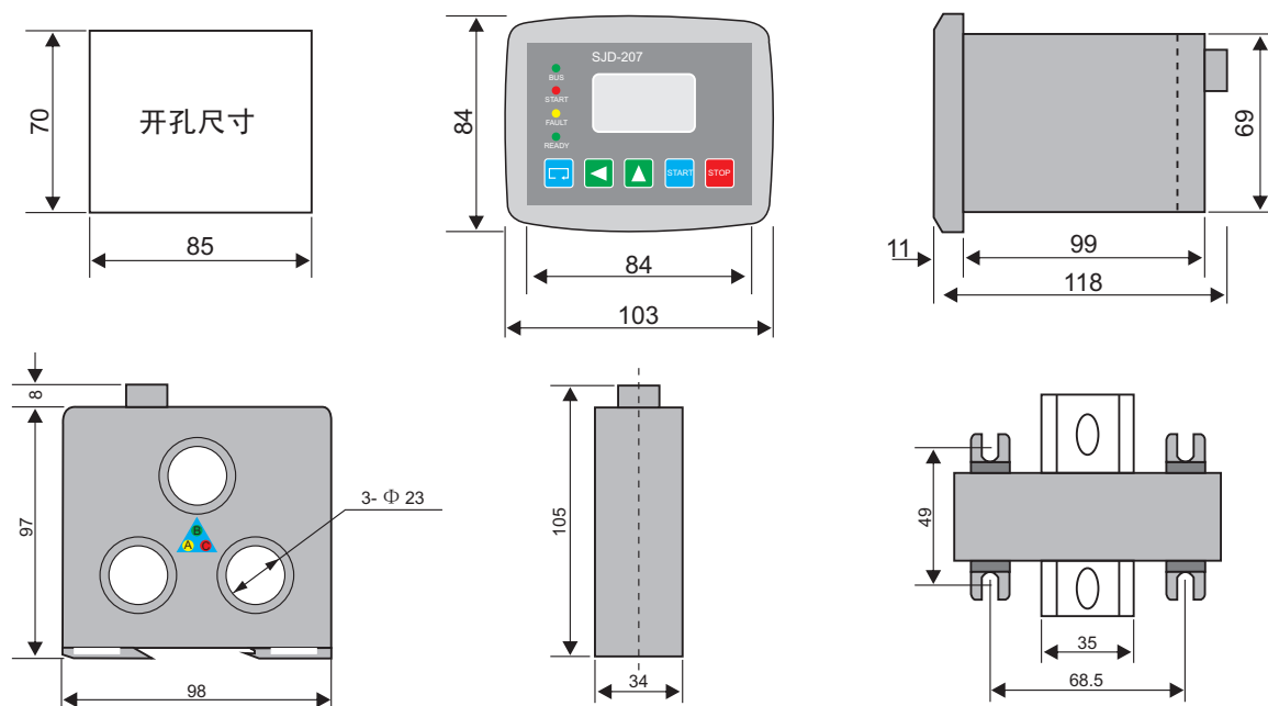
图3 SJD-207的外形尺寸
